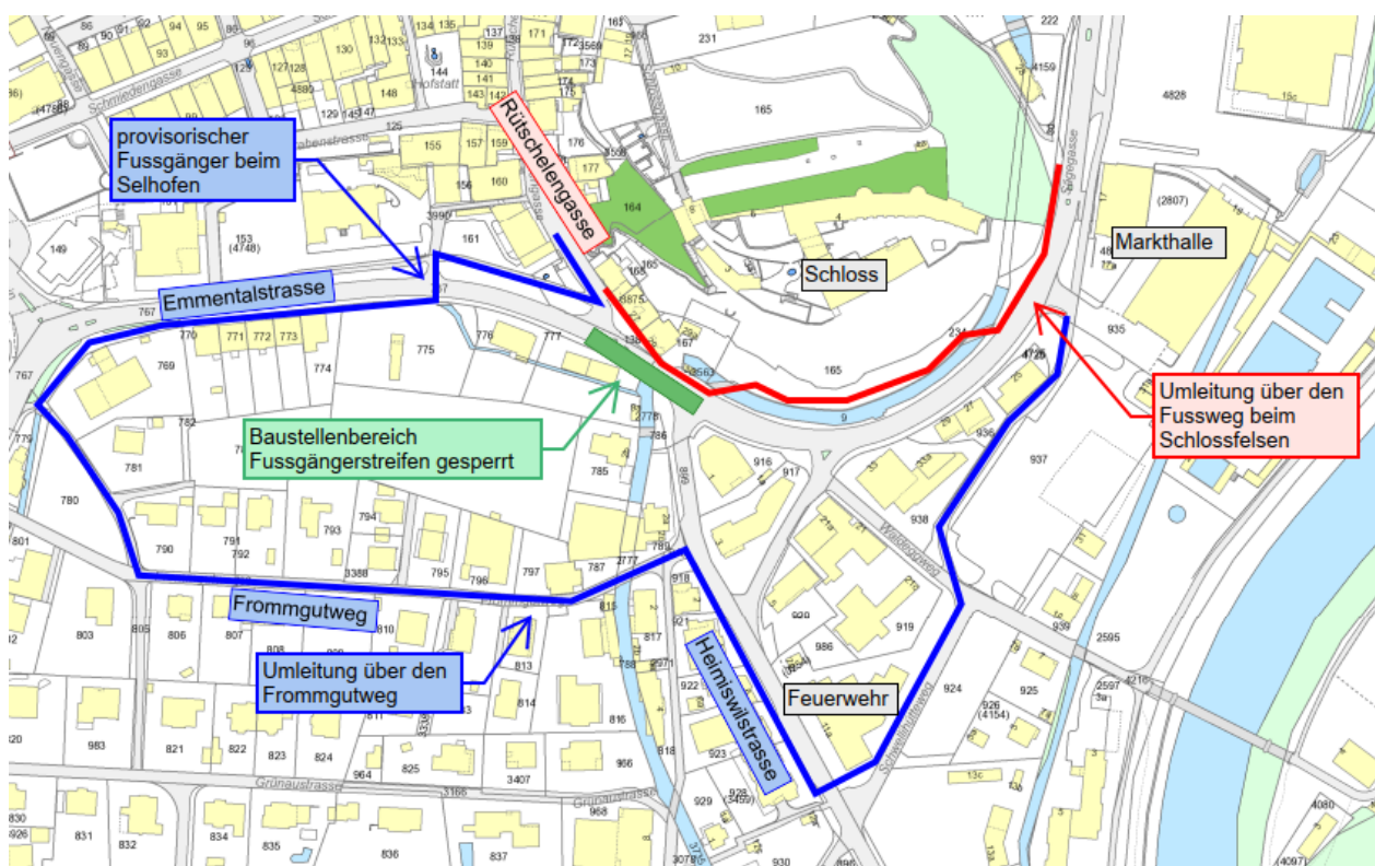
Abbildung 1: Übersichtsplan Fussgängerumleitung Emmentalstrasse.
