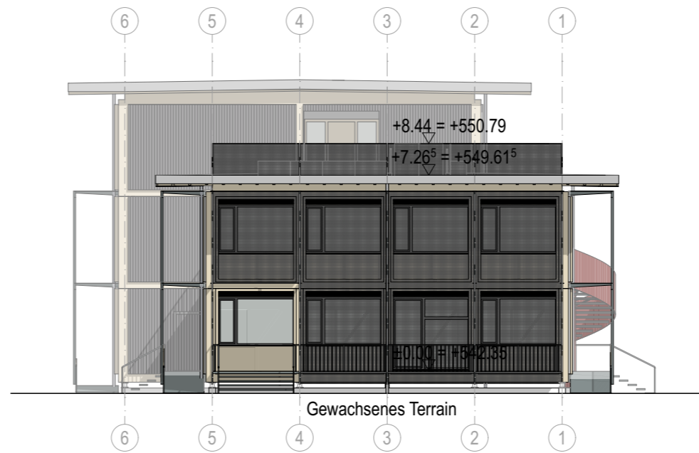
Ostfassade
